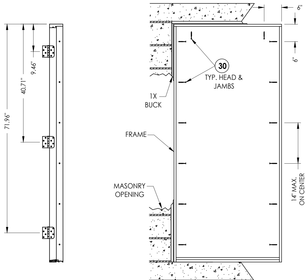
HINGE JAMB
