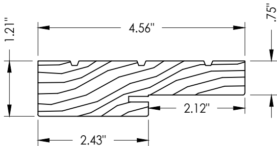
12 JAMB
